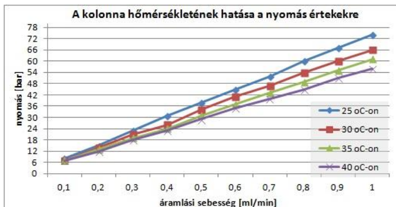
1. ábra: Kationágon a kolonna hőmérsékletének hatása a nyomás értékekre (körülmények: kolonna: CS12; eluens: 11 mmol/l H 2 SO 4 ; áramlási sebesség: 0,1-1ml/min; detektor hőmérséklete: 25 °C, kolonna hőmérséklete 25 °C, 30 °C, 35 °C és 40 °C; CSRS szupresszor; injektált minta: 25µl) [5]
