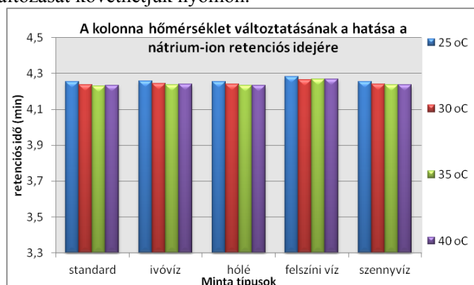
2. ábra: A kolonna hőmérsékletének hatása a nátrium-ion retenciós idejére (körülmények: kolonna: CS12; eluens: 11 mmol/l H 2 SO 4 ; áramlási sebesség: 0,1-1ml/min; detektor hőmérséklete: 25 °C, kolonna
