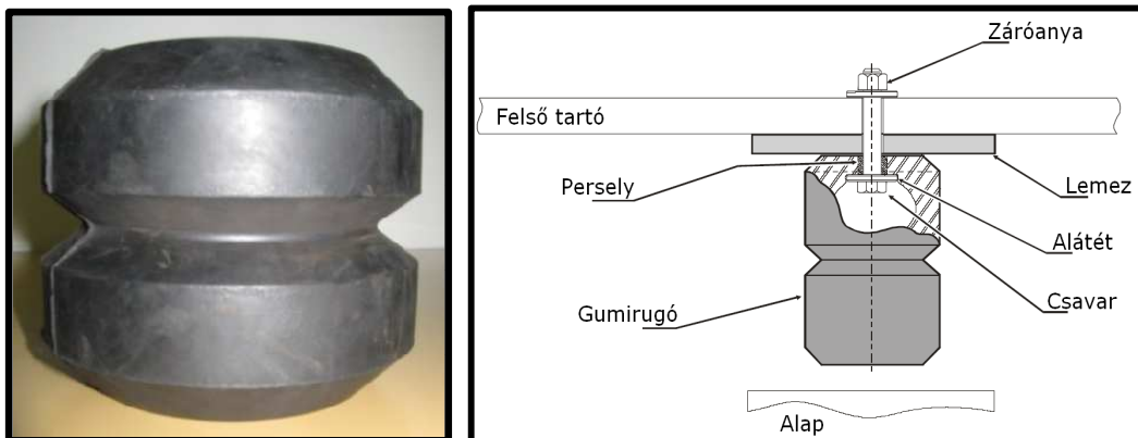
2. ábra A vizsgált gumibak és elvi beépítése
