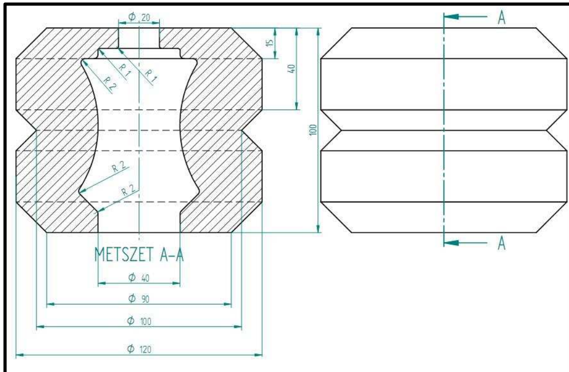
3. ábra A gumibak műhelyrajza
