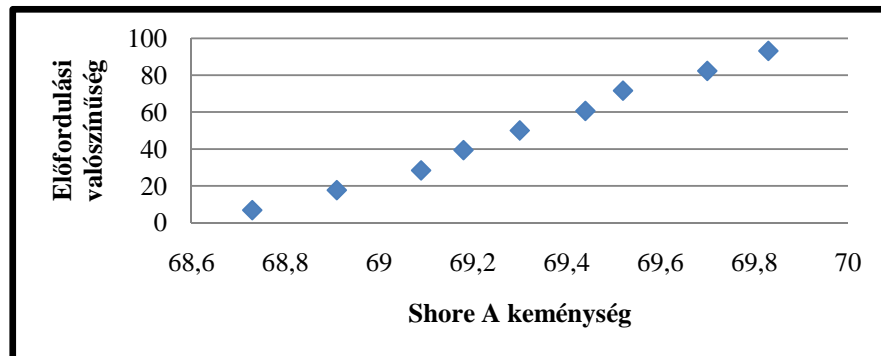
5 ábra Keménységmérési sorozat kiértékelése Gauss-papíron
