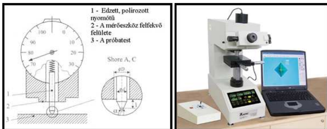
1. ábra A Shore-féle keménységmérés elve és korszerű műszere
